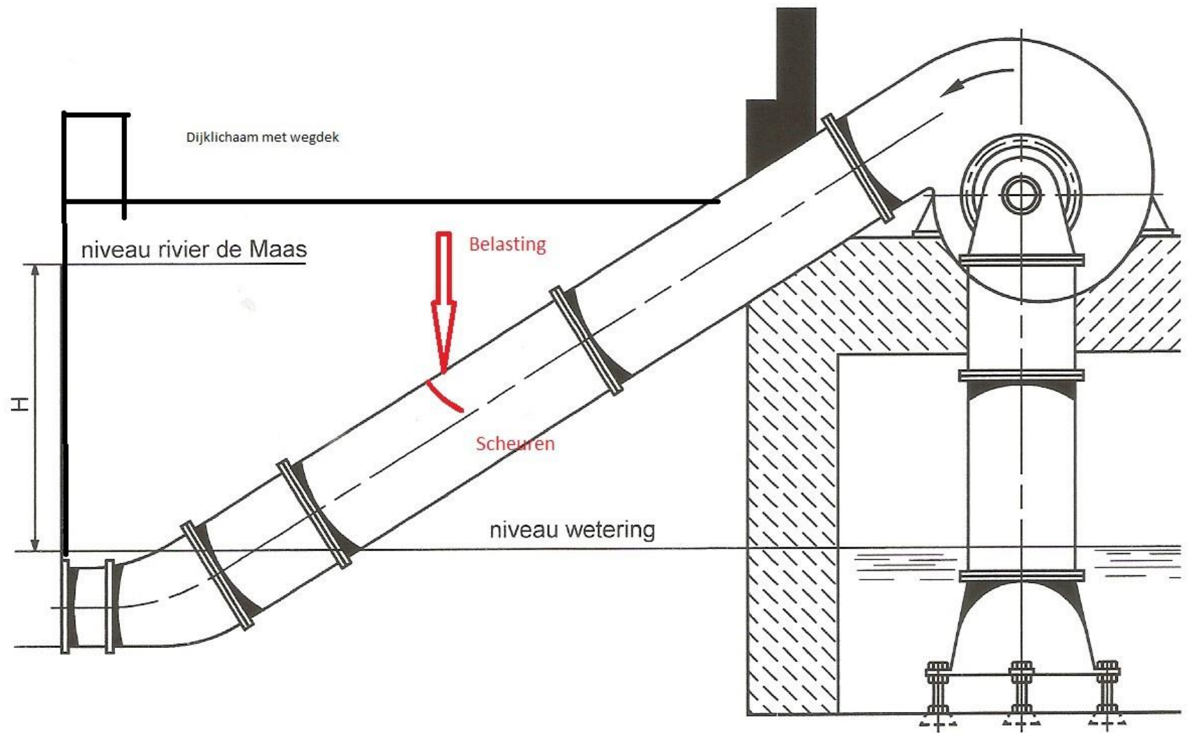
Figuur 2-84 Opvoerhoogte bemalingspomp
